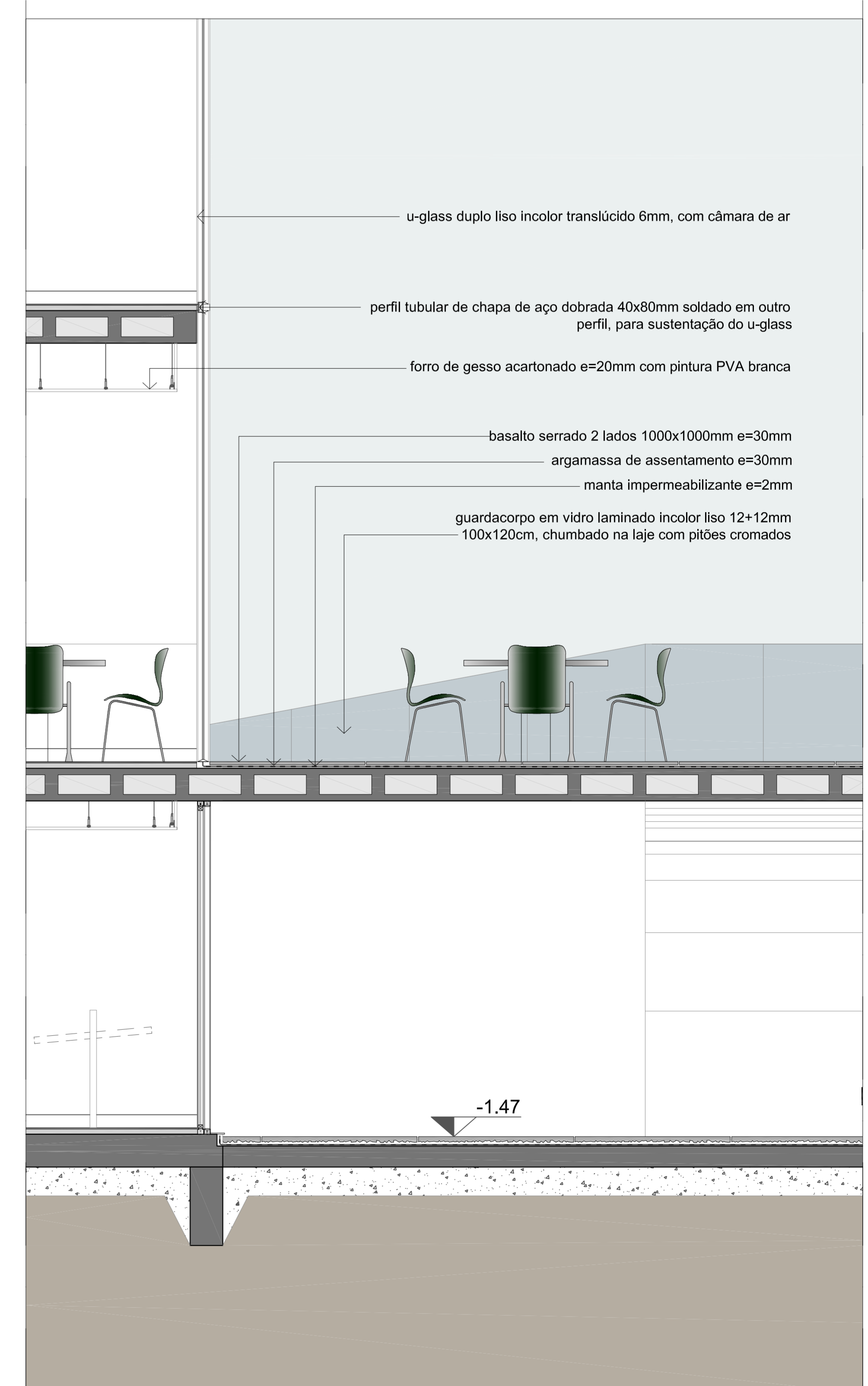
CORTE SETORIAL E=1:25
