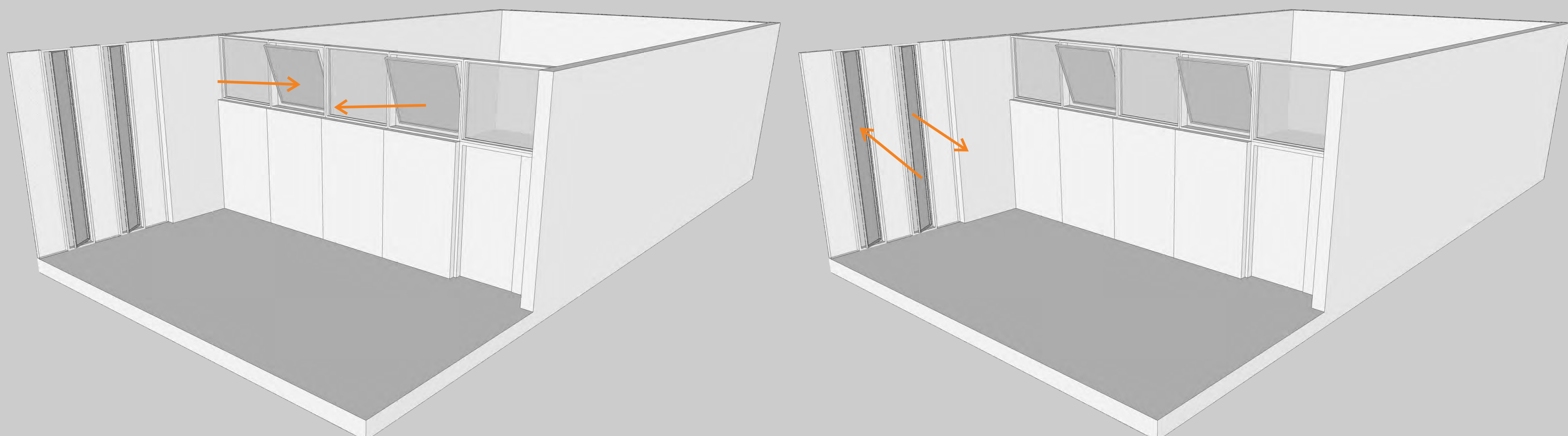
VENTILAÇÃO CRUZADA DE AR E VENTILAÇÃO CRUZADA COM A FACHADA INTERNA E EXTERNA DAS SALAS DE AULA
