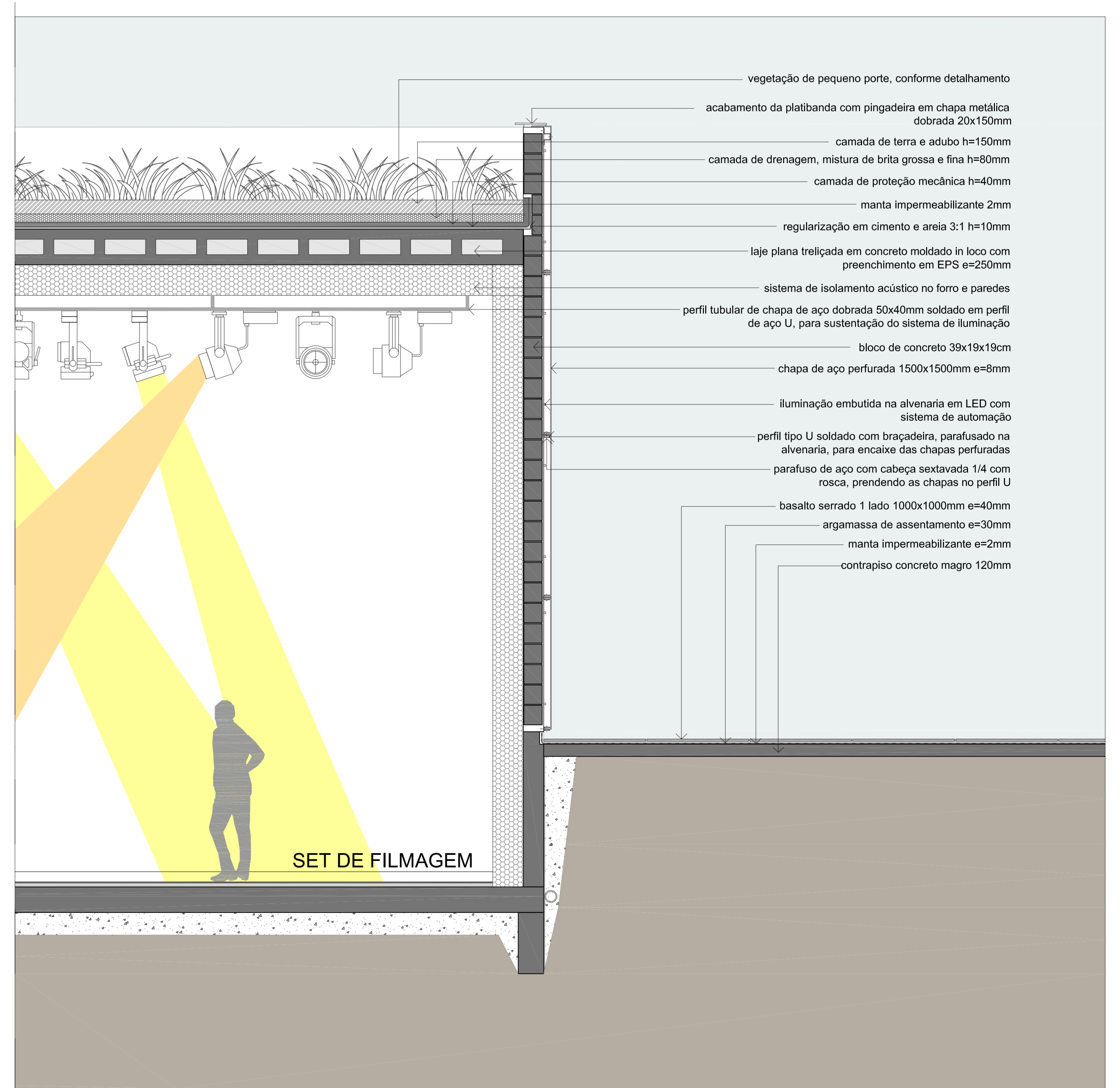
CORTE SETORIAL E=1:25
