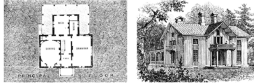
FIGURA 16 | Casa de campo. Em Cottage residences , Estados Unidos, A. J. Downing, 1844. Fonte: ACKERMAN, 1997, p. 293.
