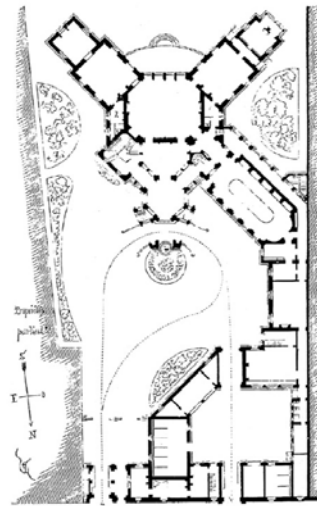
FIGURA 14 | Hôtel particulier com planta borboleta. Em Entretien 17, França. Viollet-le-Duc. Fonte: COLOUHOON, 1986, p. 167.
