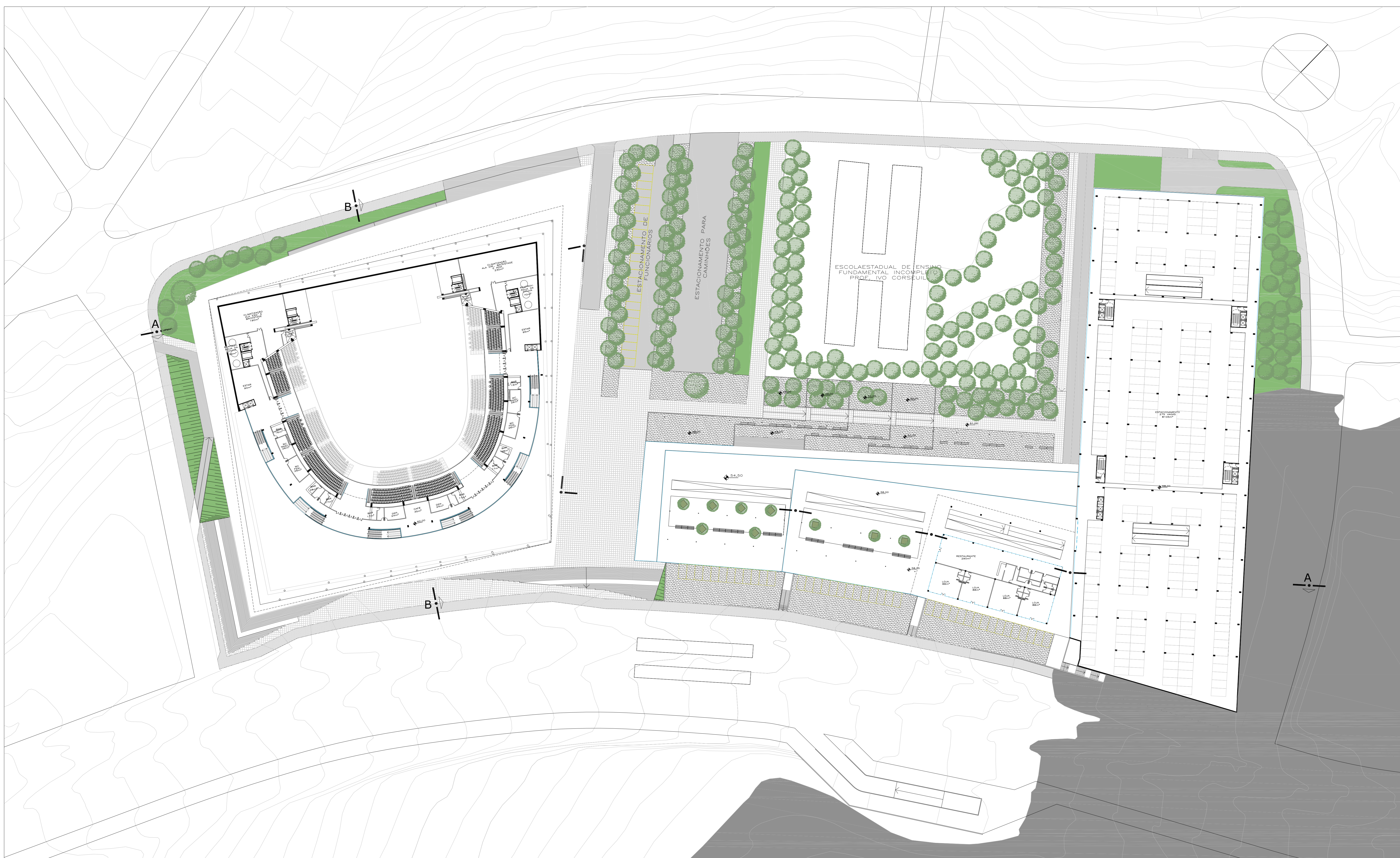
ARENA - NÍVEL 4 ESTACIONAMENTO - NÍVEL 5 LOJAS, RESTAURANTE ESC. 1:500
