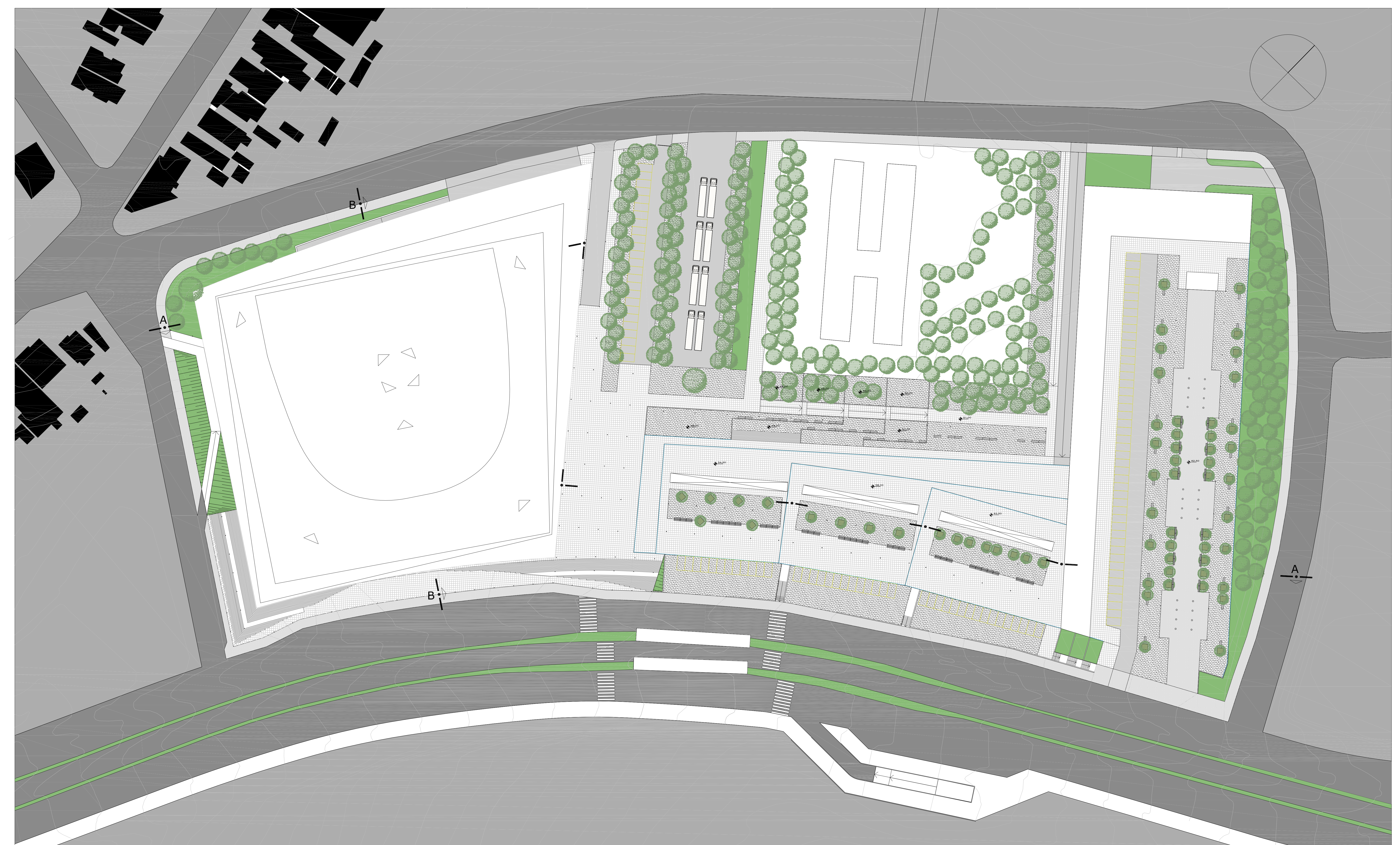
IMPLANTAÇÃO ESC. 1:500
