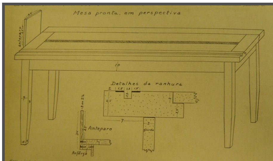
Imagem 8: Antropômetro Viola-Áureo Moraes. Fonte: Moraes, 1937, p.29.
