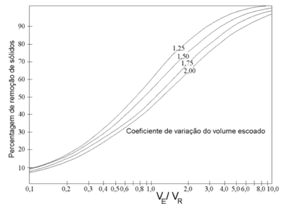
Figura 3 - Desempenho médio de longo prazo de uma bacia de detenção sob condições estáticas (adaptado de Driscoll et al., 1986).
