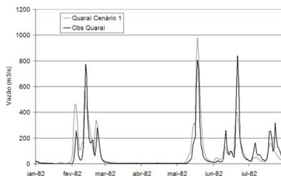
Figura 9 - Hidrogramas calculado (cinza) e observado (preto) em Quaraí/Artigas, durante o período de calibração do modelo hidrológico.
