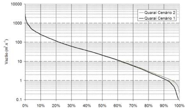
Figura 14 - Curvas de permanência de vazões do rio Quaraí junto à cidade de Quaraí, no cenário 1 (situação atual, com açudes e retiradas de água) e cenário 2 (vazão natural, sem açudes e sem retiradas de água).
