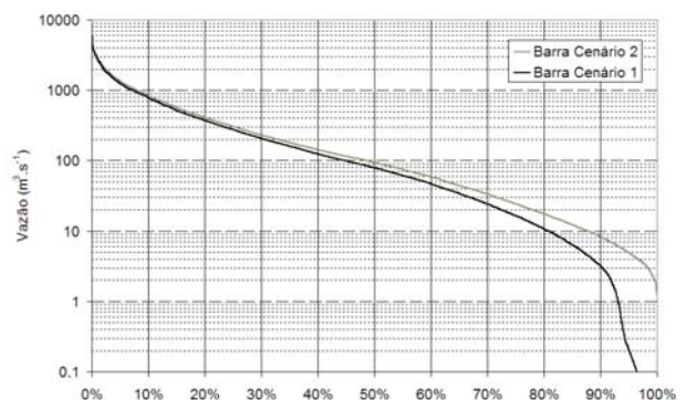
Figura 15 - Curvas de permanência de vazões do rio Quaraí na foz, em Barra do Quaraí, no cenário 1 (situação atual, com açudes e retiradas de água) e cenário 2 (vazão natural, sem açudes e sem retiradas de água).
