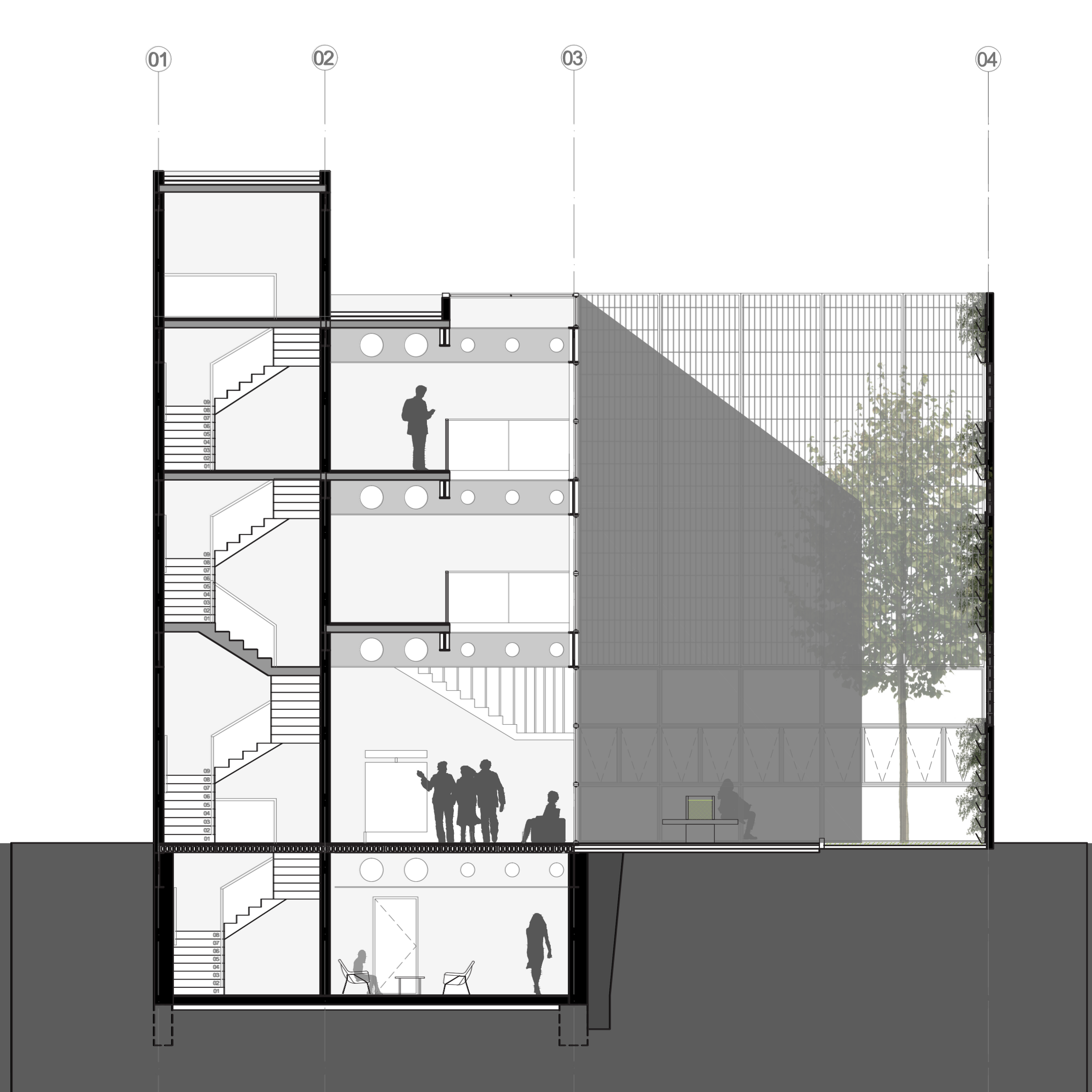
Corte DD' | 1:75
