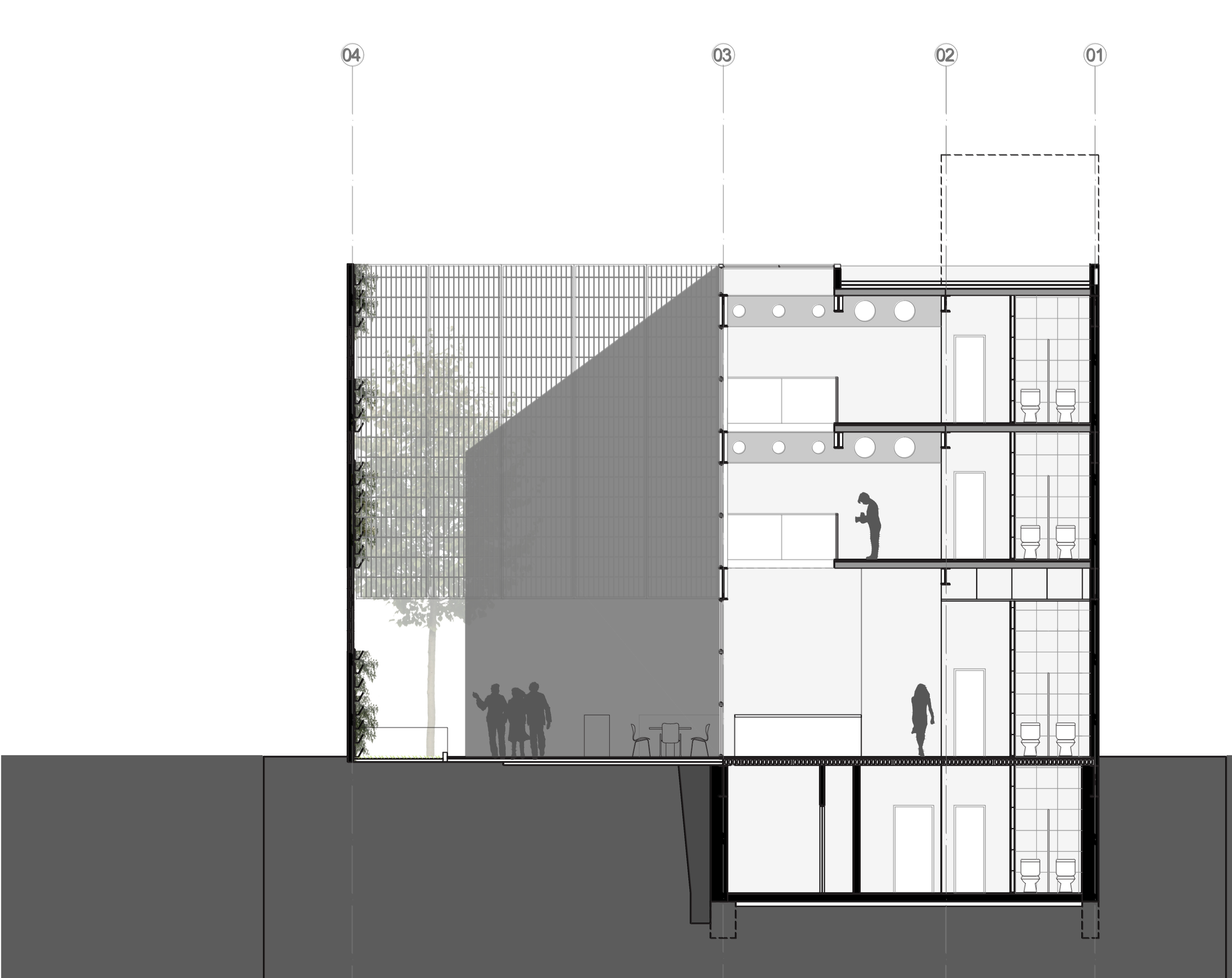
Corte CC' | 1:75
