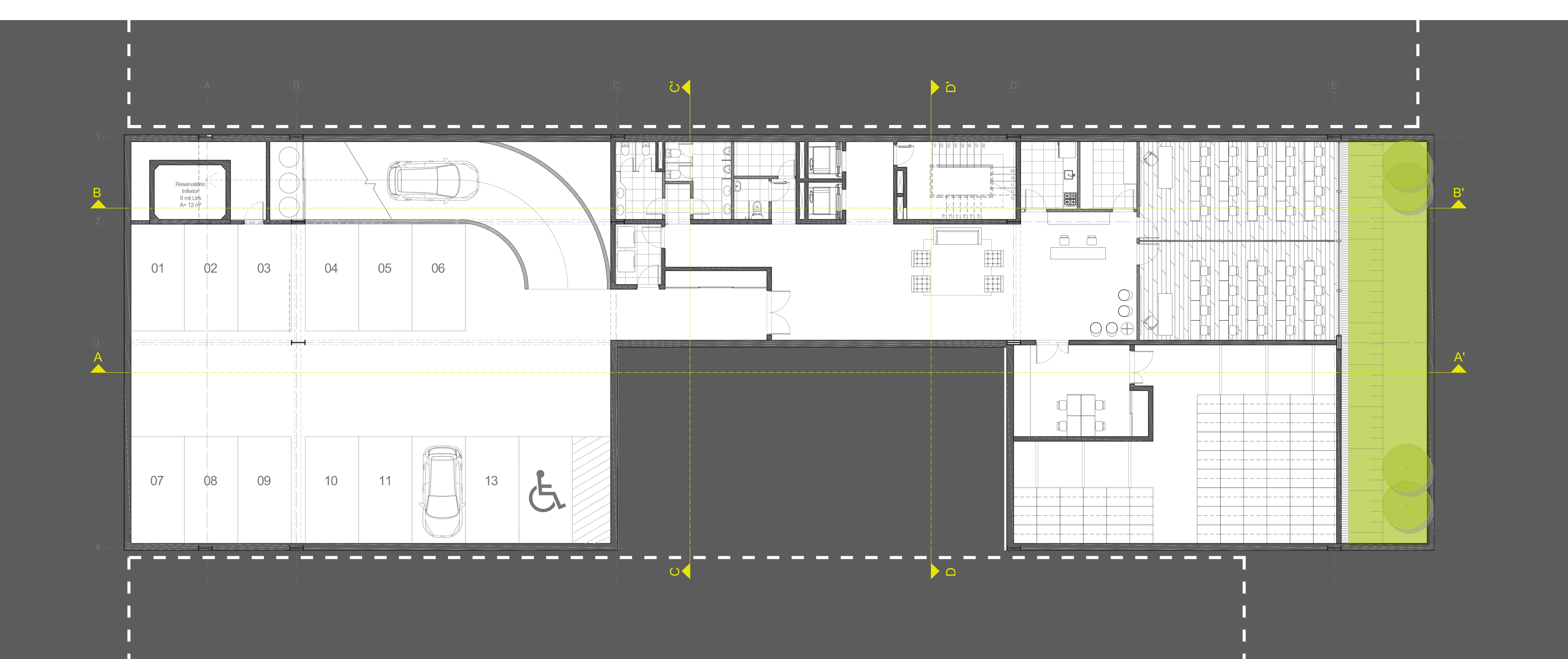
Planta Baixa Subsolo | 1:75
