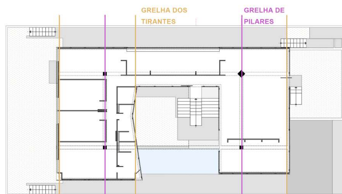
SEGUNDO PAVIMENTO ESC: 1/200
