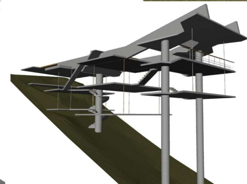
PERSPECTIVA ESTRUTURAL
