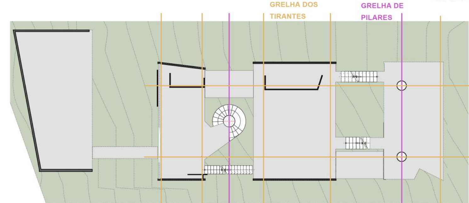
PAVIMENTO INTERMEDIÁRIO ESC: 1/200
