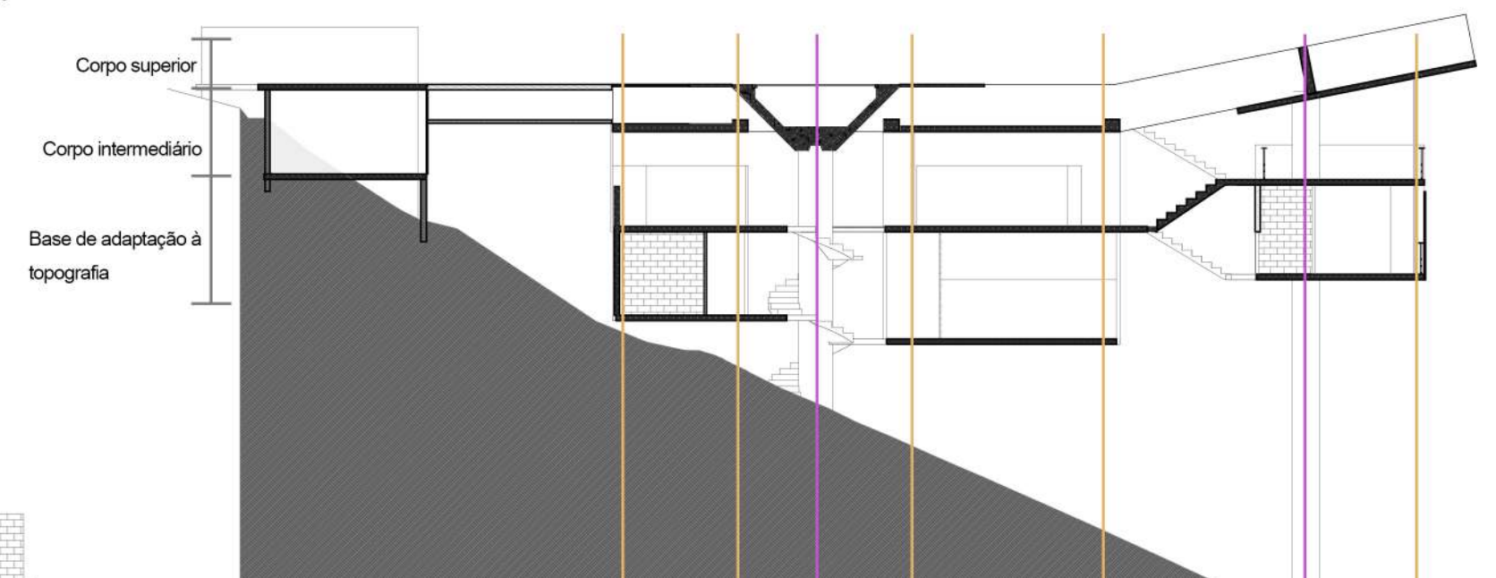
CORTE LONGITUDINAL ESC: 1/200
