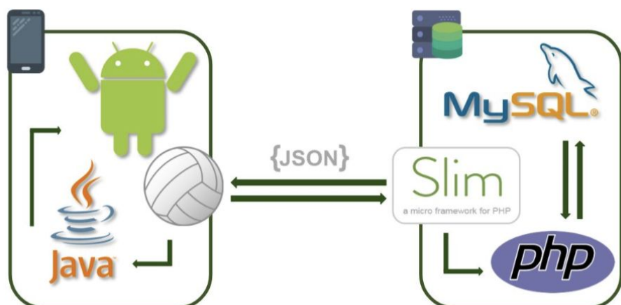
Figura 1. Arquitetura do aplicativo e serviços externos
