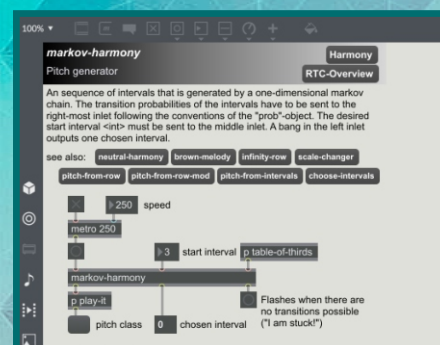
ALGORITMO GERADOR DE NOTAS DA BIBLIOTECA RTC-LIB
