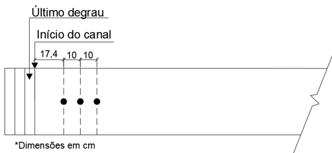
Figura 5.- Posições de medições das pressões médias ao longo de bacia de dissipação.
