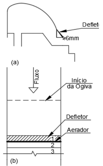
Figura 4.- a) vista lateral e b) vista superior de vertedouro em degraus com aerador e defletor
