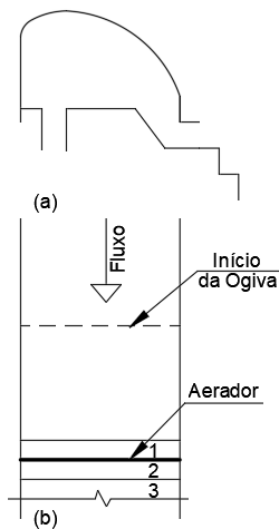
Figura 3.- a) vista lateral e b) vista superior de vertedouro em degraus com aerador
