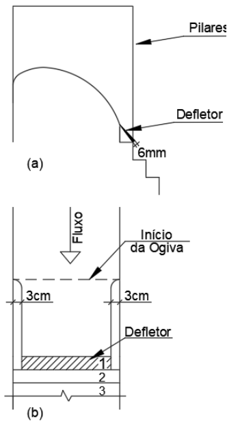
Figura 2.- a) vista lateral e b) vista superior de vertedouro em degraus com pilares e defletor
