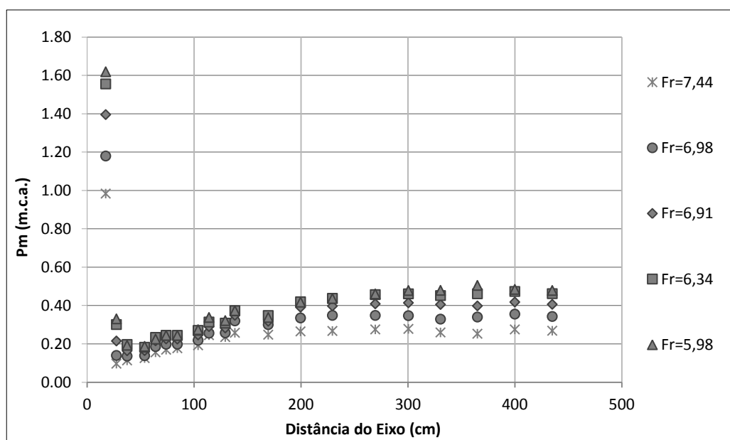
Figura 1.- Pressões médias ao longo de bacia de dissipação a jusante de calha em degraus obtidas por Novakoski et. al (2017)
