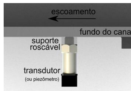
Figura 6.- Instalação dos transdutores para medição de pressões médias ao longo da bacia de dissipação.
