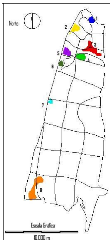
Figura 5. 40 – Zonas de ocorrência do cisne-do-pescoço-preto no Banhado do Taim/RS para fins de identificação do histórico de longo período do índice de adequabilidade
