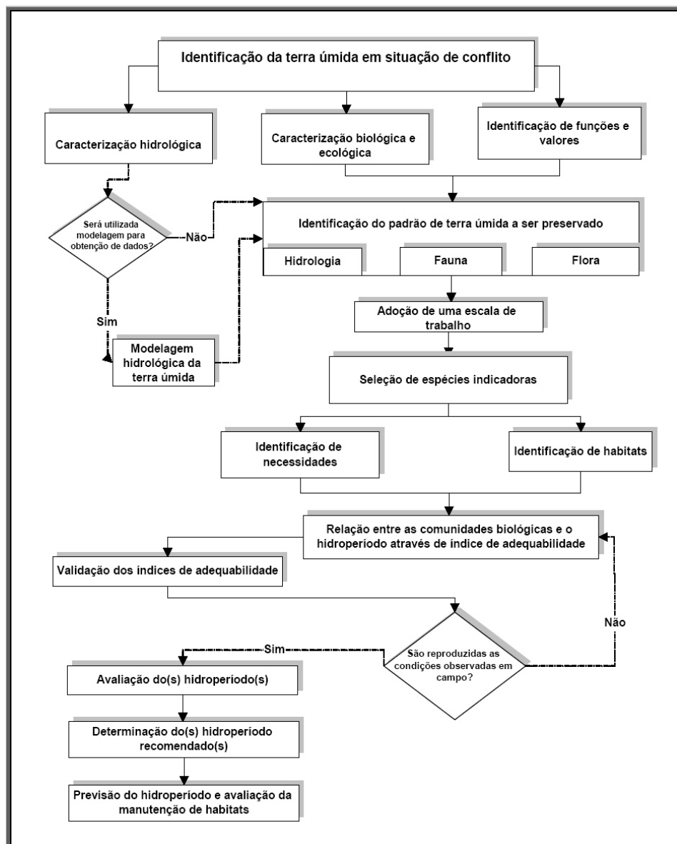
Figura 3. 1 – Fluxograma da seqüência metodológica
