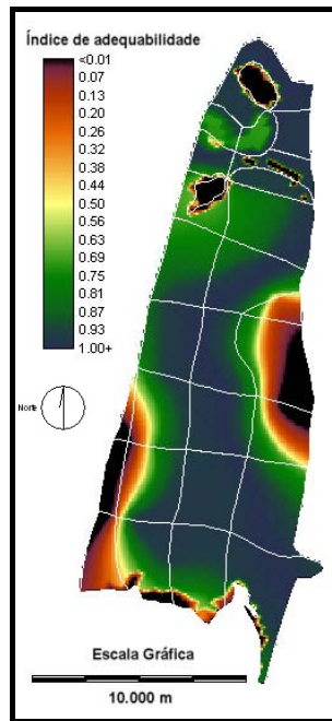
Figura 5. 21– Exemplo do produto da análise do índice de adequabilidade da Zizaniopsis bonariensis no interior do Banhado do Taim/RS
